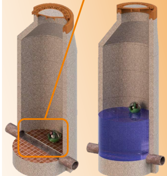
Einbaudarstellung
